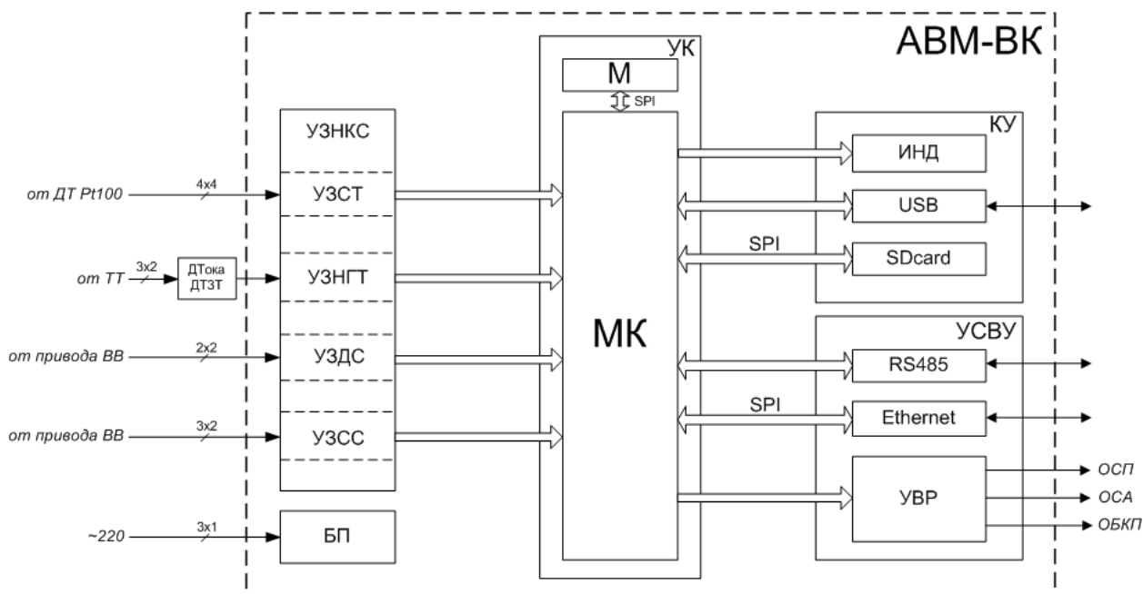
Рис. 5 – Функциональная схема АВМ-ВК
