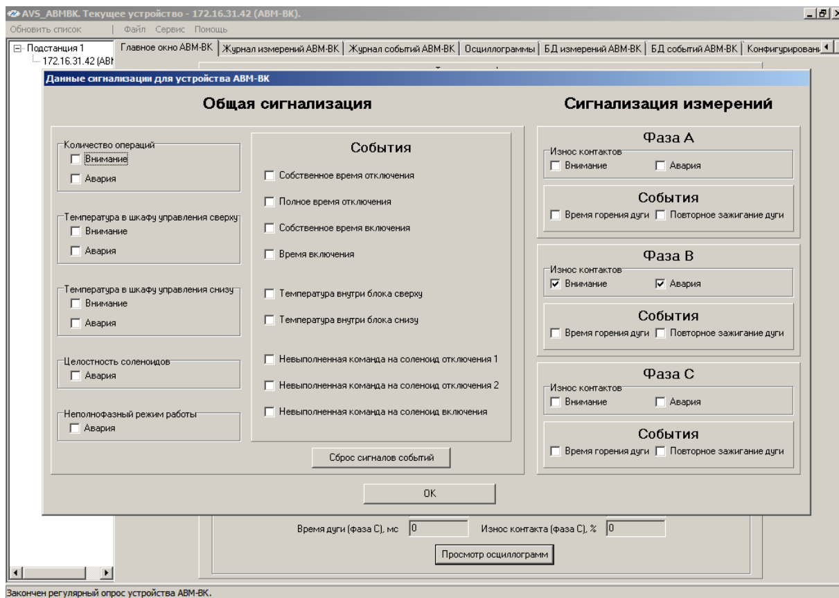
Рис. 12 – Экраны программы AVS_ABMBK – окно «Данные сигнализации»
