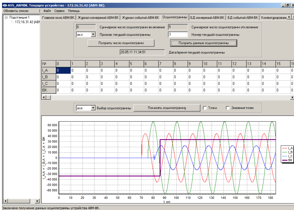
Рис. 16– Экраны программы AVS_ABMBK – вкладка «Осциллограммы»
