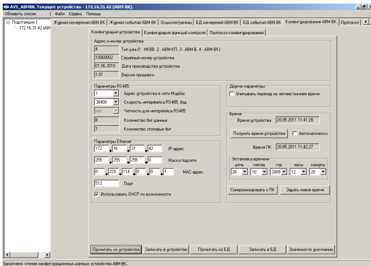
Рис. 9 – Экраны программы AVS_ABMBK – вкладка «Конфигурация устройства»
