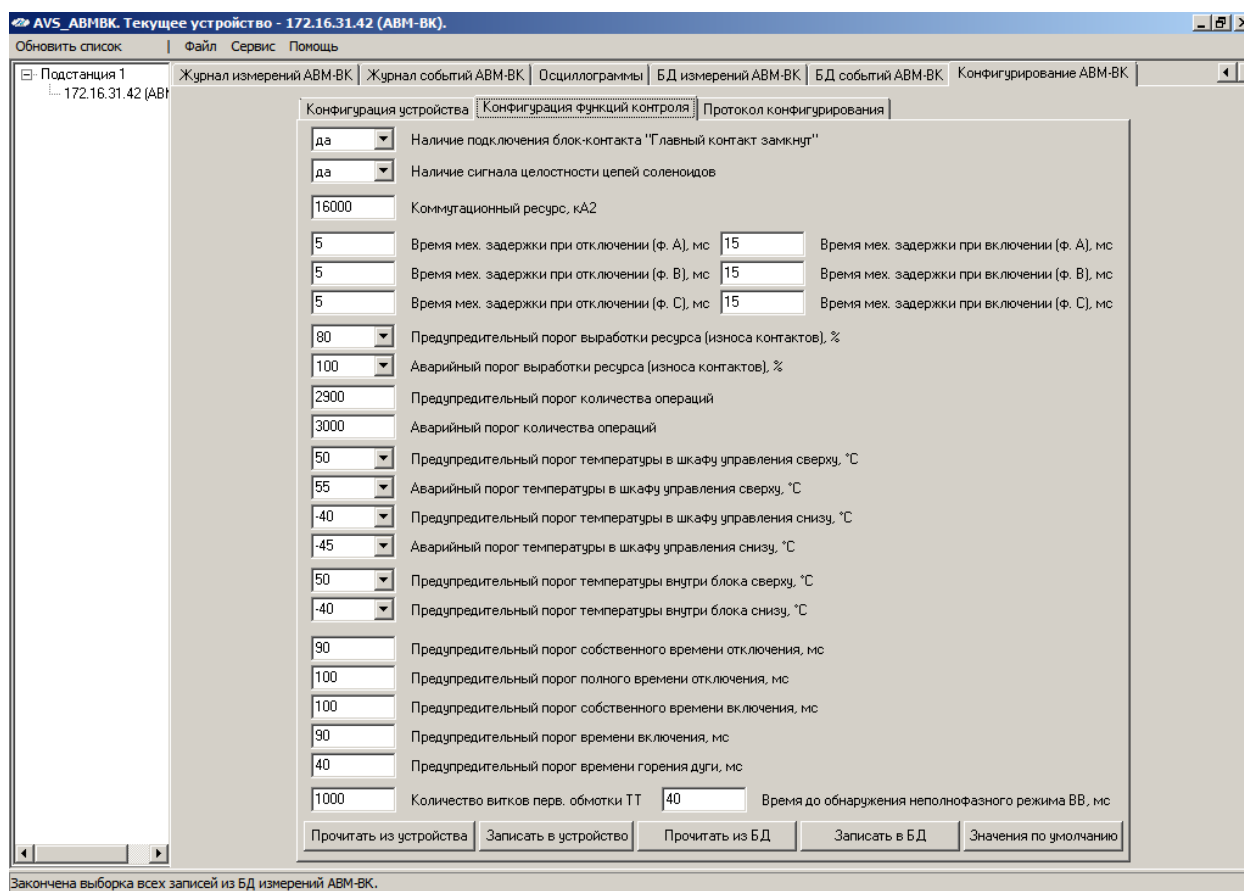
Рис. 10 – Экраны программы AVS_ABMBK – вкладка «Конфигурация функций контроля» для вкладки «Конфигурирование АВМ-ВК»
