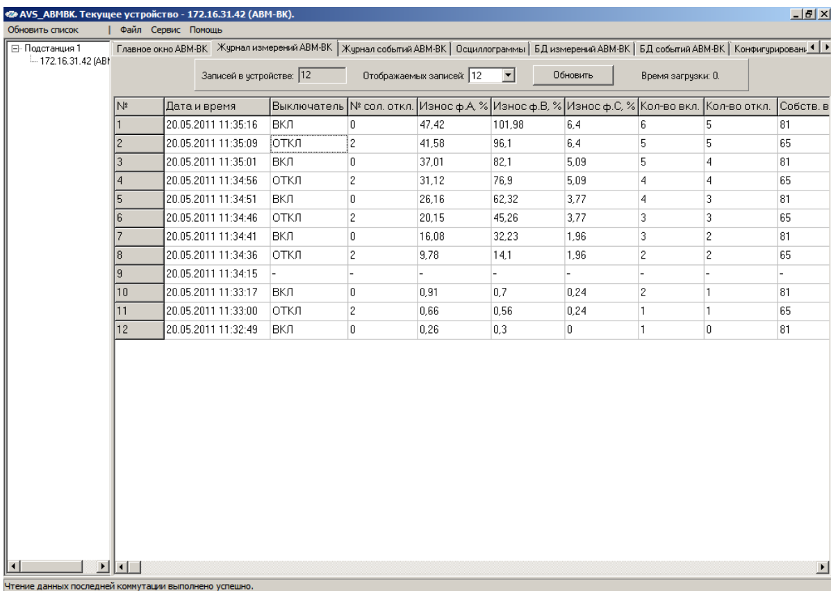
Рис. 15 – Экраны программы AVS_ABMBK – вкладка «Журнал измерений АВМ-ВК»
