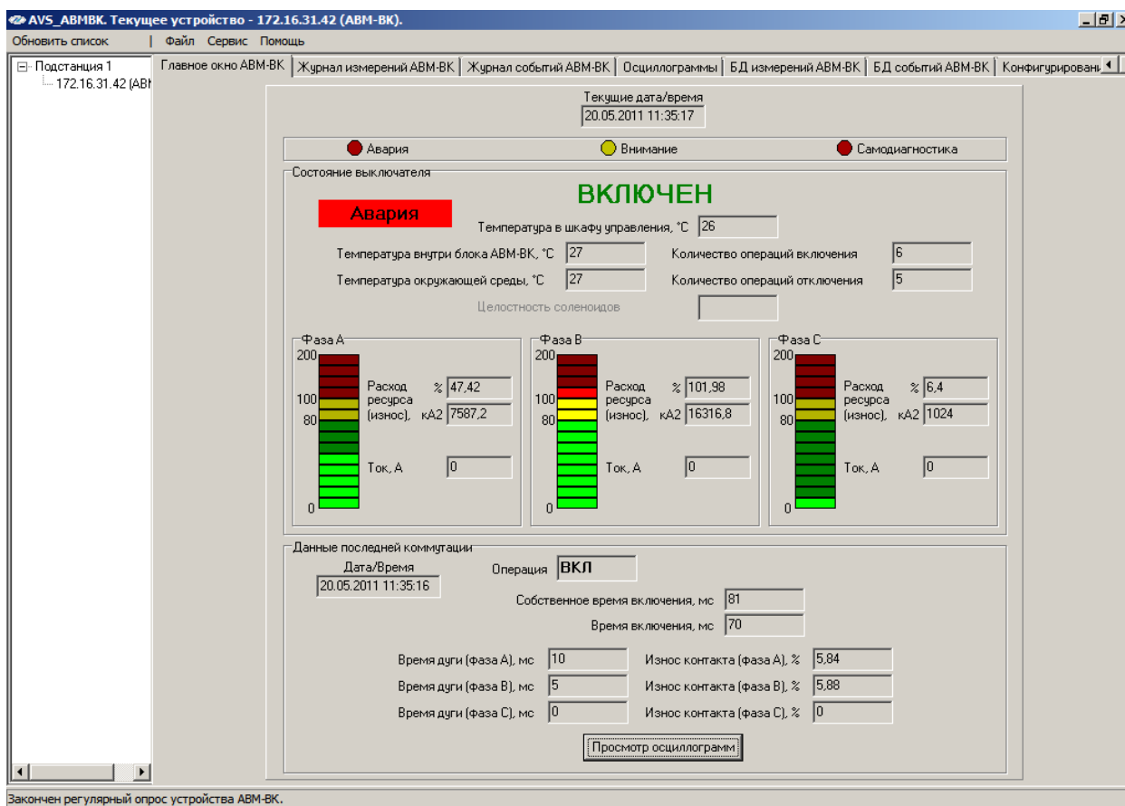
Рис. 11 – Экраны программы AVS_ABMBK – вкладка «Главное окно АВМ-ВК»
