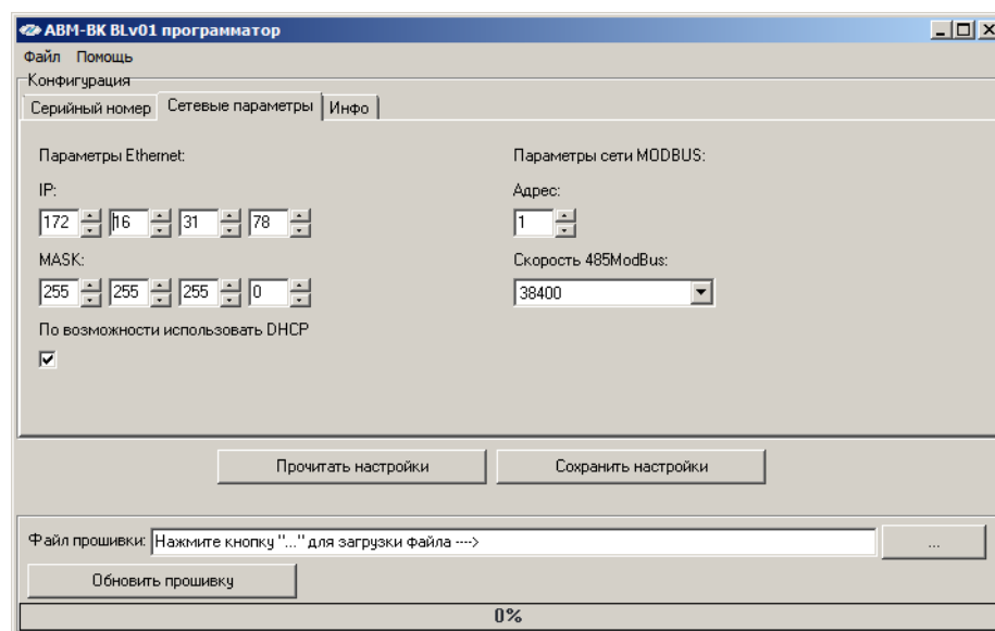
Рис. 8 - Вкладка "Сетевые параметры"
