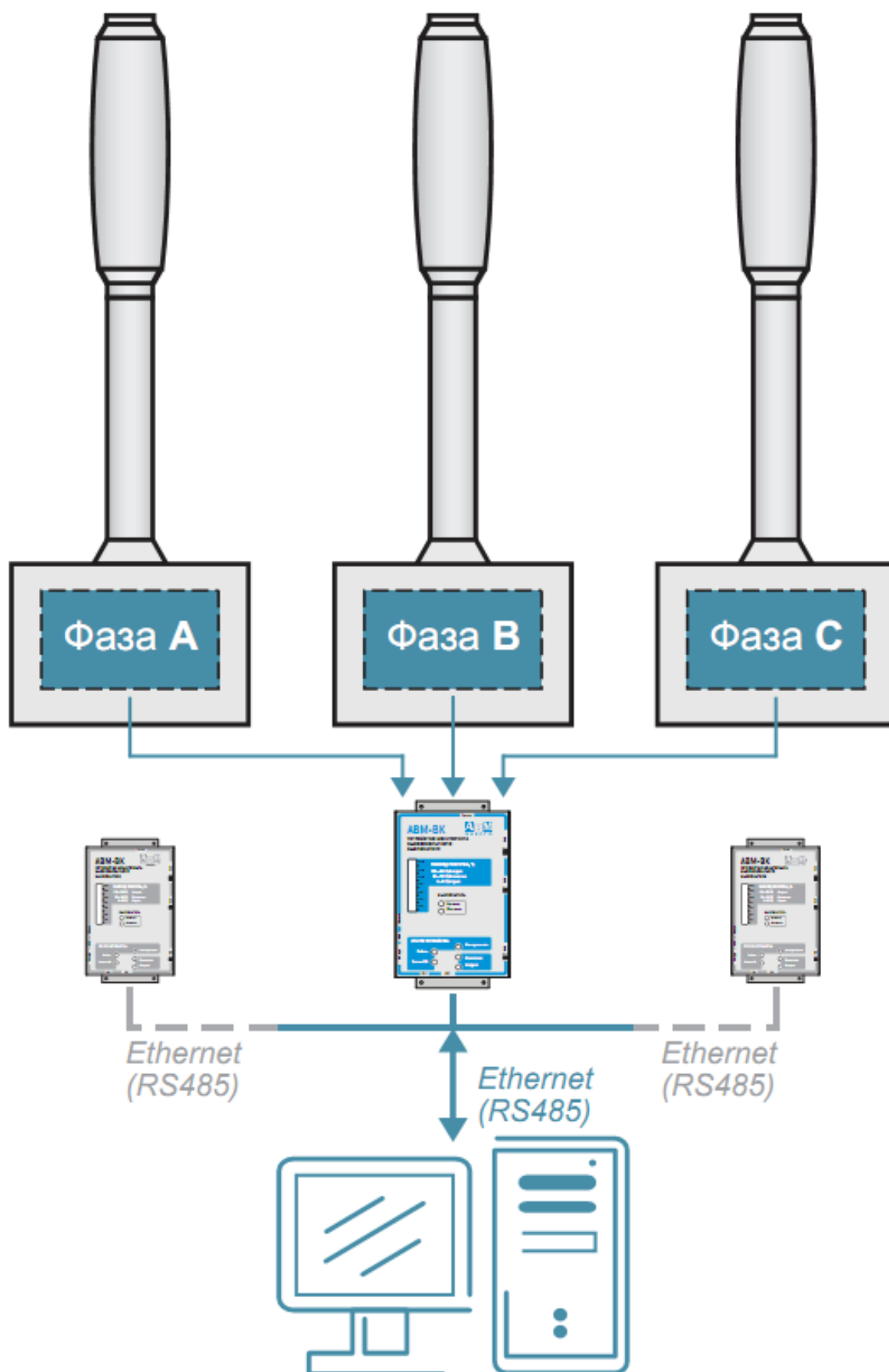
Рис. 1 – Иерархическая система мониторинга выключателей энергообъекта
